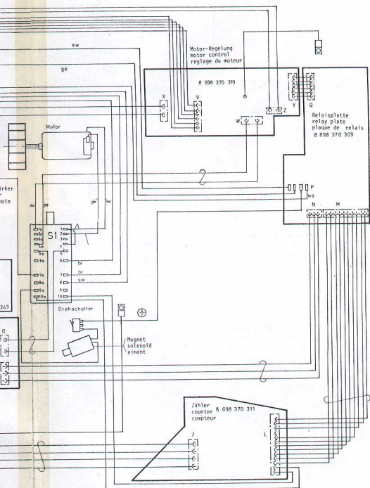
Verdrahtungsplan wiring diagram plan de câblage 8 699 976 618 (10 78-VKD1)
